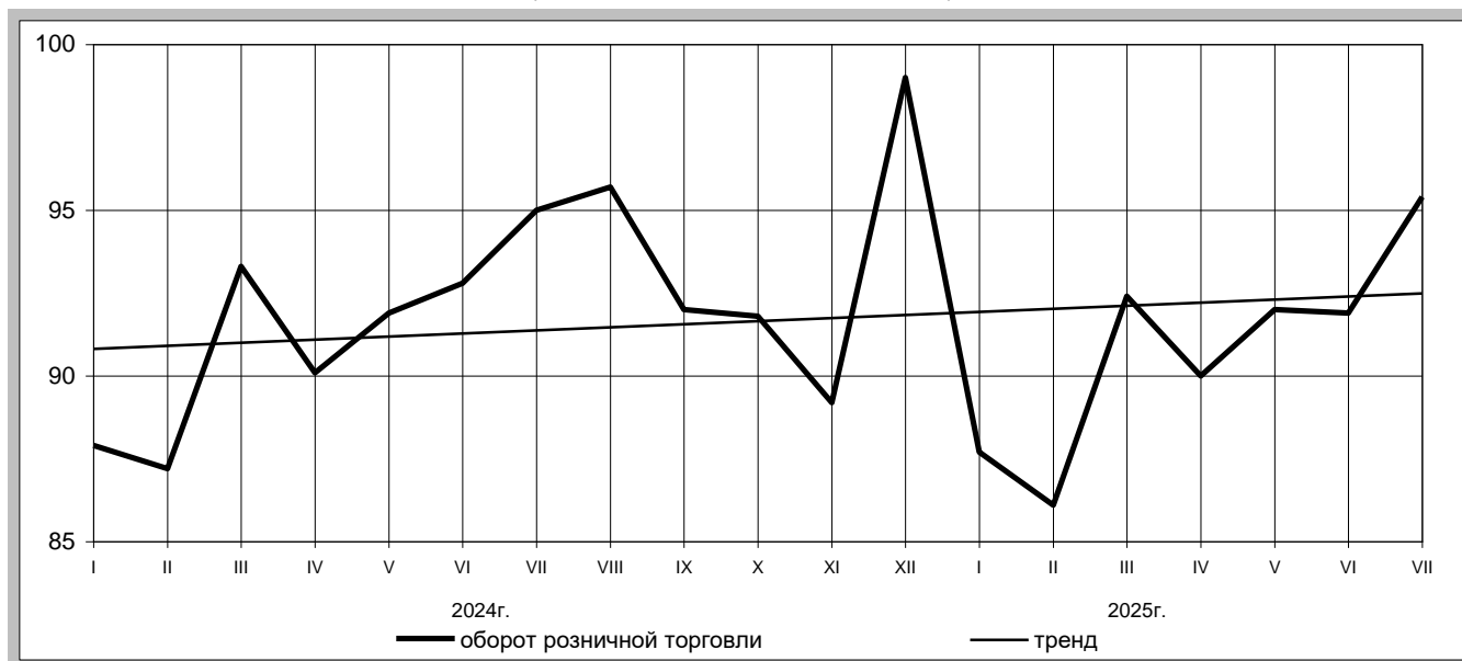
Динамика оборота розничной торговли (в процентах к декабрю 2023 года)
